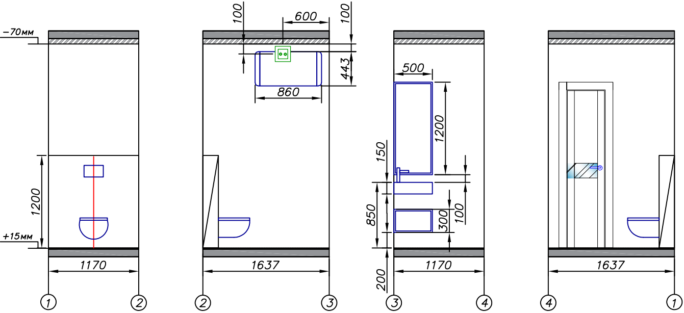
Развертка стен санузел.
