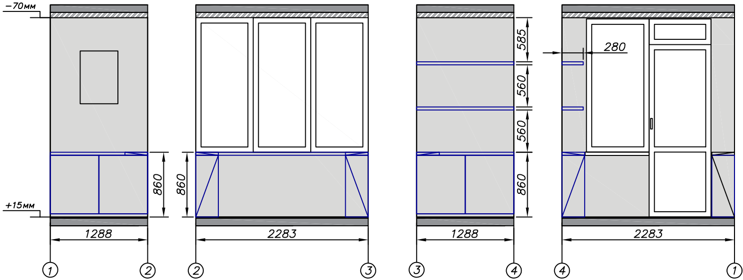
Развертка стен балкон.
