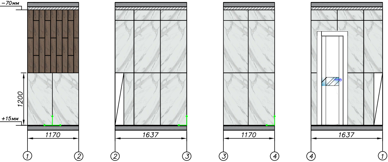
Развертка стен санузел.
