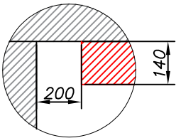
Узел 2 Ниша для штор
