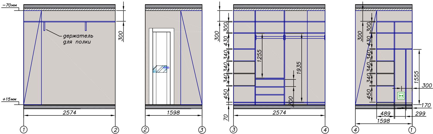
Развертка стен гардероб.
